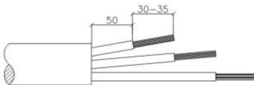
Рисунок 6. Оголение электрокабеля
